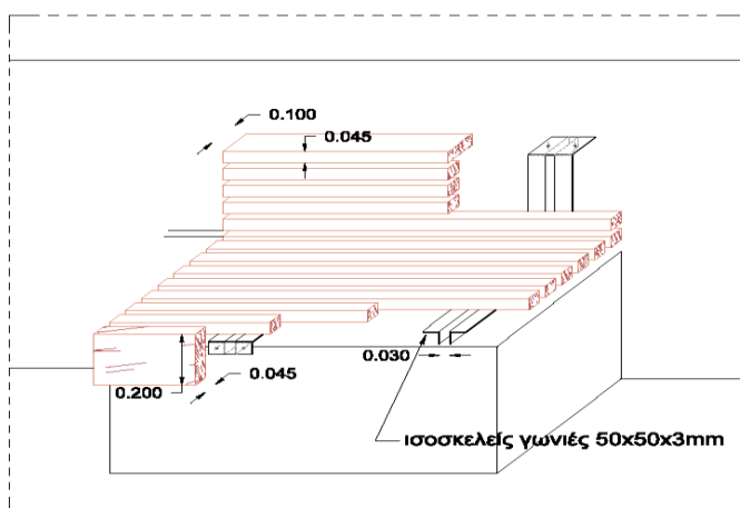
Σχέδιο λεπτομέρειας 1
