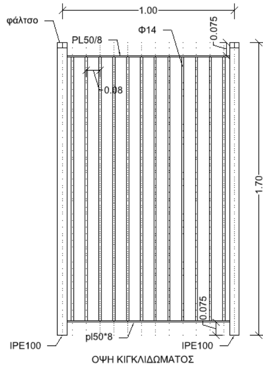
ΣΧΕΔΙΟ ΚΙΓΚΛΙΑΔΩΜΑΤΟΣ
